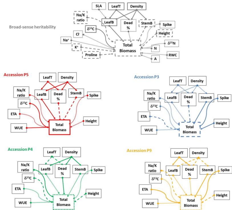
Figura: Heredabilidad en sentido amplio (H 2 ) del germoplasma en variables morfoagronómicas, fisiológicas e isotópicas. Relaciones entre variables que mostraron diferencias entre accesiones (P3, P4, P5, P9) en condiciones de sequía y salinidad. Valores relativos: ____ alto, _ _ _ medio, ..... bajo (en línea gris para H 2 , en líneas de color para accesiones). Densidad de macollos (Density), longitud de hojas por macollos (LeafT), biomasa de hojas verdes (LeafB), biomasa de tallos verdes (StemB), porcentaje de tejidos muertos (Dead%), altura de la planta (Height), evapotranspiración acumulada (ETA), eficiencia en el uso del agua (WUE), proporción de macollos con espigas (Spike%), isótopos de 13C ( \delta^{13}C ), isótopos de 15N ( \delta^{15}N ), contenido relativo de agua (RWC), tasa fotosintética neta (A) y concentración de prolina (proline).
